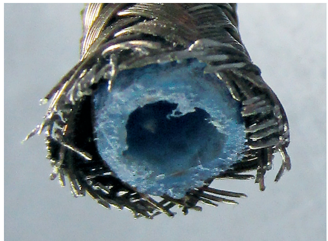
ADDINOL Cliptec XHS Serie – Schmierstoffzuleitung ohne Ablagerungen, voll durchgängig / ADDINOL Cliptec XHS series – Feed pipes without de- posits, full functional capability
