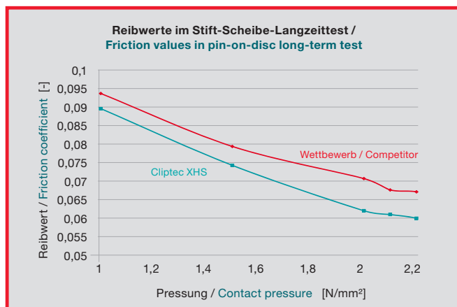
Grafik 2: Reibwerte für ADDINOL Cliptec XHS im Stift-Scheibe-Langzeittest im Vergleich zum Wettbewerb – Deutliche Reduktion von Temperatur und Verbrauch dank Minimierung des Reibwertes
