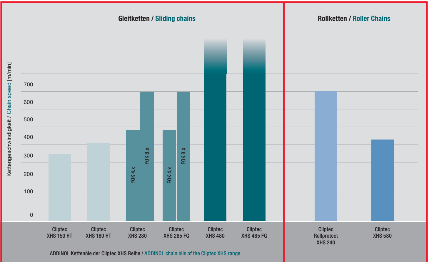
Grafik 1: Einsatzbereiche in Folienreckanlagen verschiedener Generationen mit niedrigen, mittleren und hohen Reckgeschwindigkeiten
