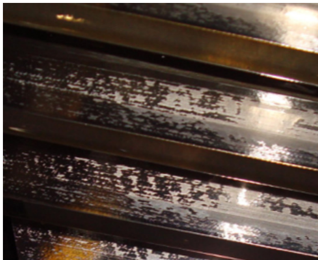
Bild 2: Starke Zunahme der Oberflächenschädigung durch Wettbewerbsöl im parallel laufenden Extrudergetriebe.
