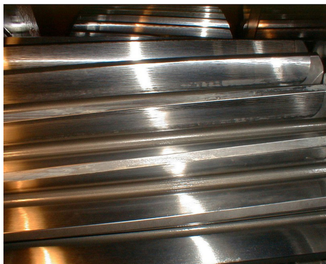
Bild 1: Eco Gear stoppt erfolgreich Micro-Pitting Wachstum. Das Öl verhindert größere Schäden und verlängert die Lebensdauer des Getriebes deutlich.
